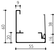
cód. 4140 Perfi base de AL con apertura a presión
