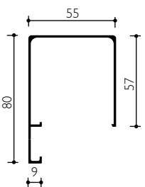
cód. 4045 Perfil superior y lateral en AL
